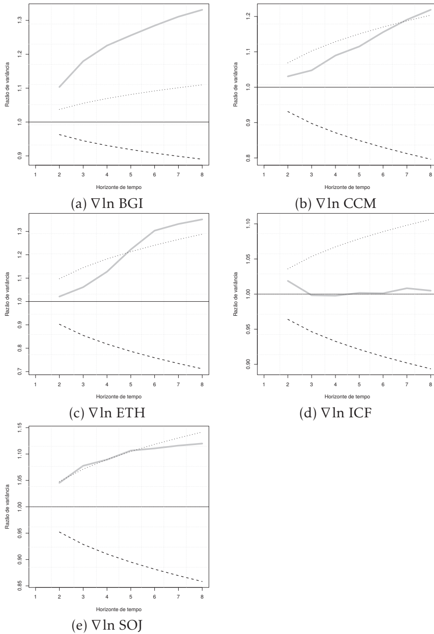
Figura 1: Razões de variância
