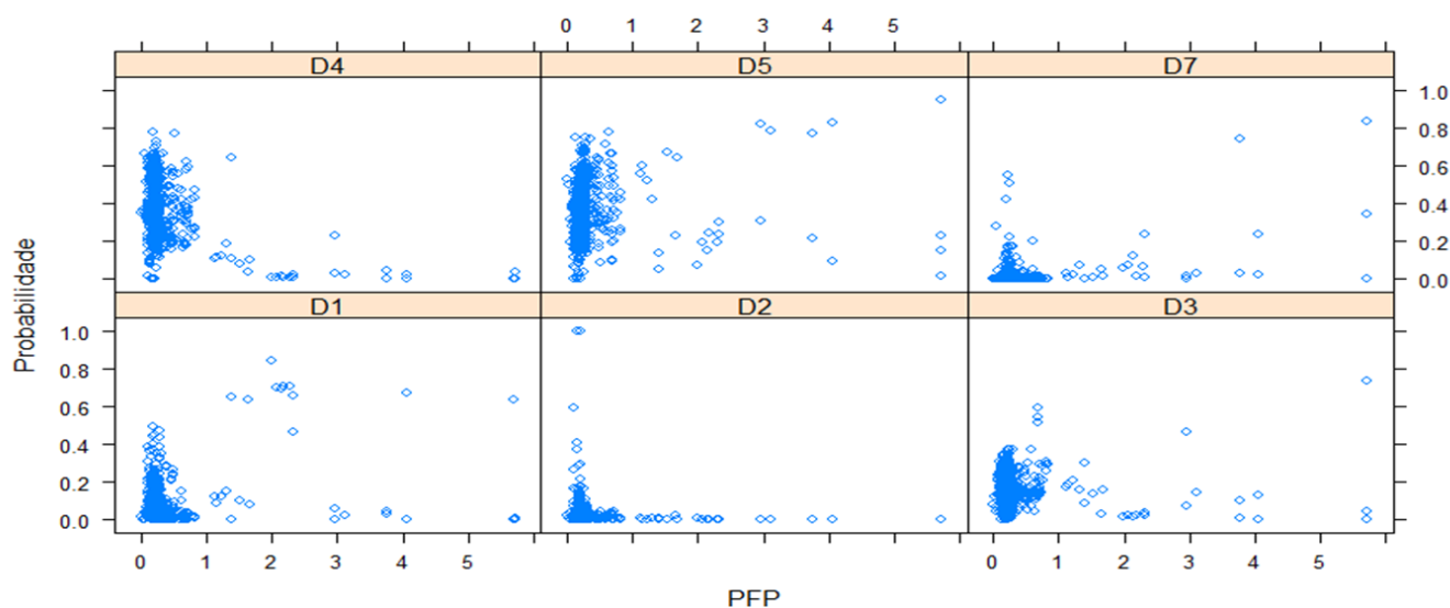
Figura 1 Probabilidade de escolha de categoria \times PFP
