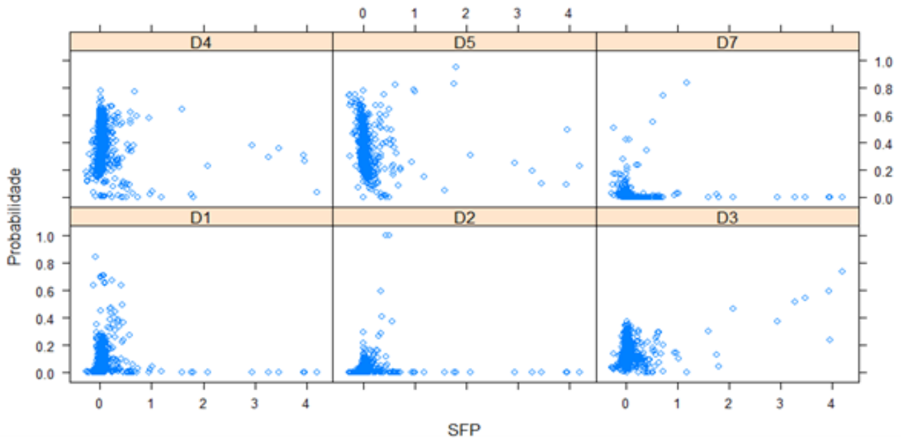
Figura 2 Probabilidade de escolha de categoria \times SFP
