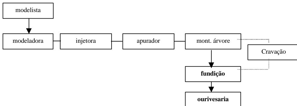
Figura 1 – Fluxograma da produção de peças
